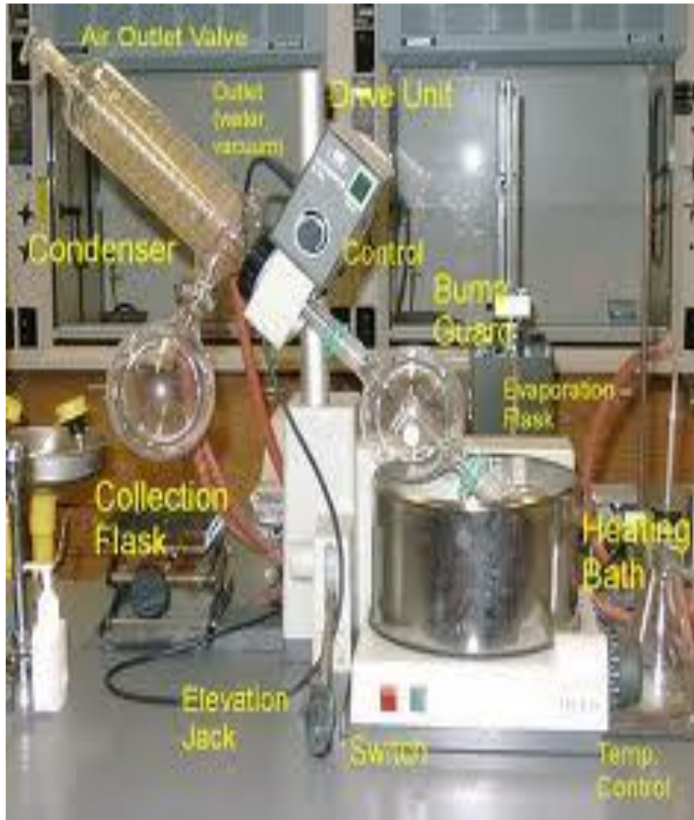
Rotatory evaporator
